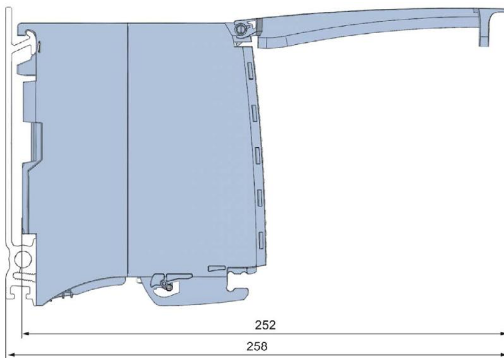
Рисунок А-2 Габаритный чертеж модуля DI 16x24VDC BA вид сбоку, с открытой передней крышкой
