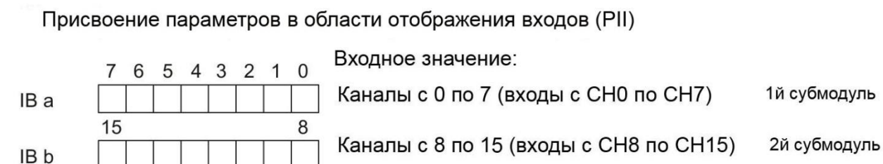
Рисунок 4-2 Пространство адресов для конфигурации модуля в режиме 2x8- канального входа DI 16x24VDC BA S
