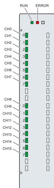
Рисунок 5-1 Светодиодные индикаторы модуля DI 16x24VDC BA
