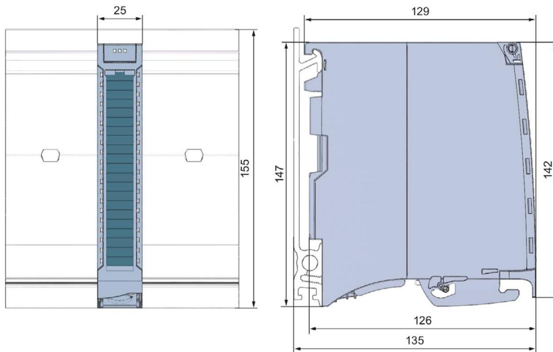
Рисунок А-1 Габаритный чертеж модуля DI 16x24VDC BA
